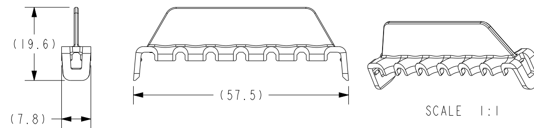
FRH-A12-T TPA - PDM, FRH
